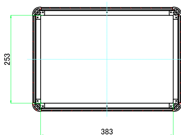
C-C ( 1 : 6.5 )
